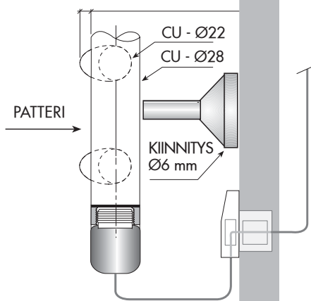
Puolikiinteä asennus
