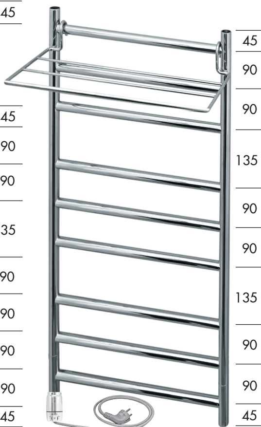
CRES-920 - 400 CRES-920 - 502
